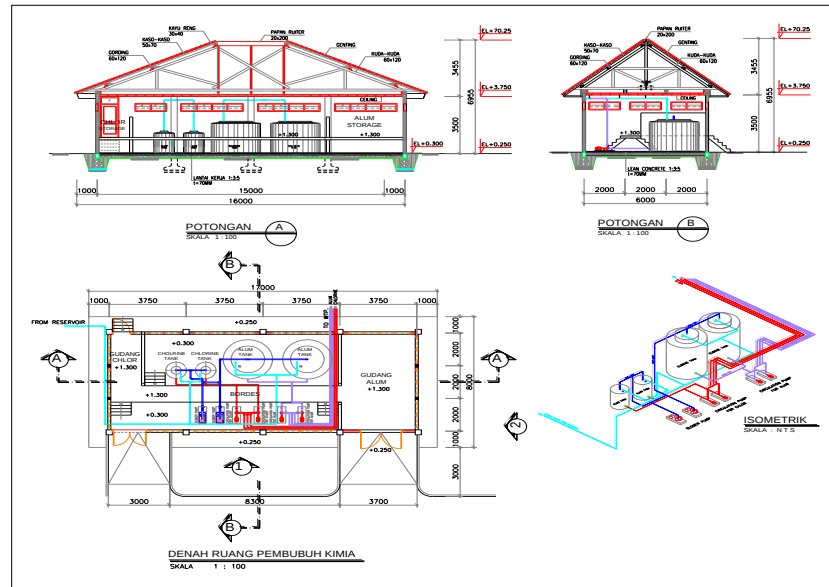
Rumah Kimia, terdiri dari ruang unit koagulasi, unit desinfeksi, unit netralisasi, unit floridasi, unit pelunak kesadahan, dan unit penghilang Fe dan Mn. Laboratorium terdiri dari ruang tes fisiokimia, tes bakteri (ruang pembiakan bakteri dan persiapan tes bakteri), tes biologi, ruang pertemuan, ruang gelap, kamar gas, tempat penyimpanan bahan kimia, dan tempat perkakas. Gudang terdiri dari gudang kimia (tempat penyimpanan koagulasi, desinfeksi, netralisasi, floridasi, pelunak kesadahan, dan penghilang Fe dan Mn) dan gudang umum (tempat penyimpanan suku cadang dan perlengkapan khusus).
