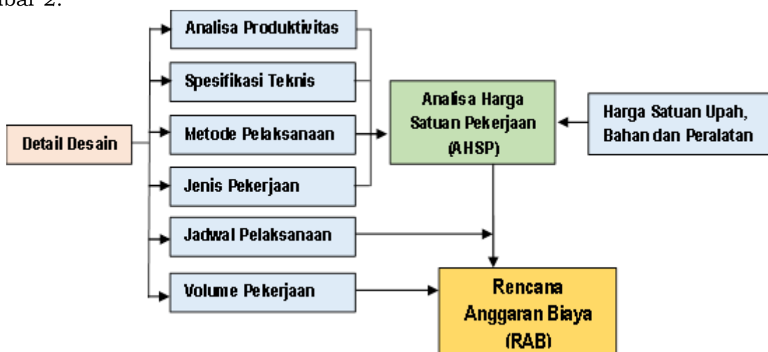
Gambar 2 Tahapan Penyusunan RAB Kegiatan Infrastruktur Pengendali Banjir
