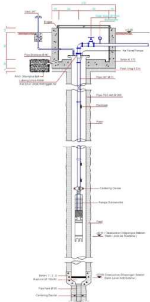
Gambar 3.3. Model Bangunan Pengambilan Air Tanah
